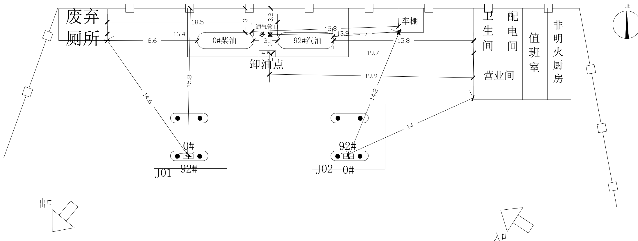
中国石化销售股份有限公司安徽安庆怀宁三桥加油站总平面现状示意图
